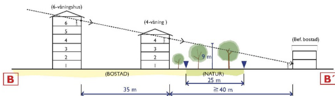
Sektionsbild B-B'
